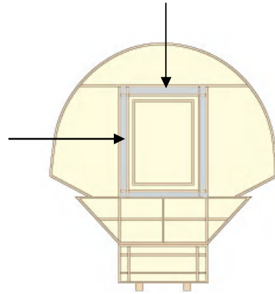
P29 扇ねふたの構造
